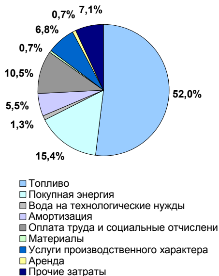
Себестоимость производства электроэнергии, %
