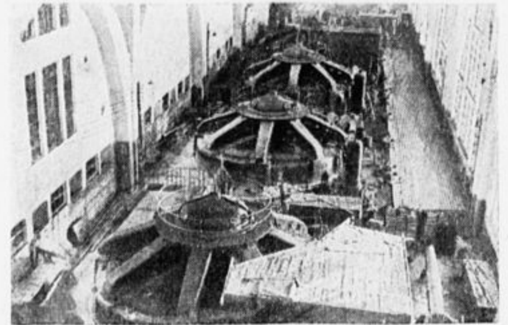
Турбинный зал главной силовой станции. На первом плане 4 шведских турбины.
